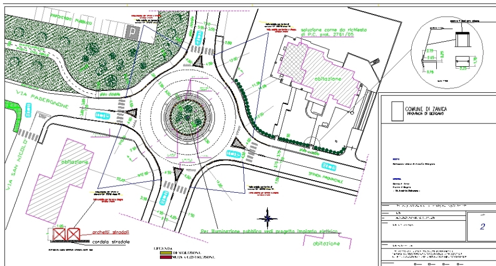
Il progetto della rotatoria
